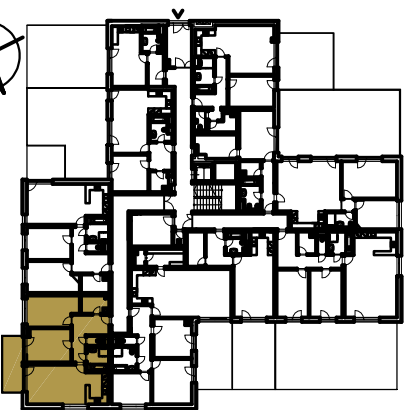
PŮDORYS PATRA 1 NP
