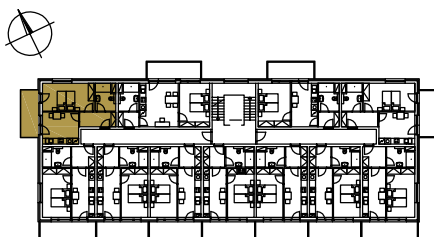
PŮDORYS PATRA
