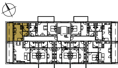
PŮDORYS PATRA
